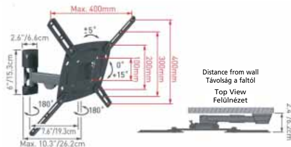
E330 LCD tv tartó 3 funkci LCD tv mount 3 functions
