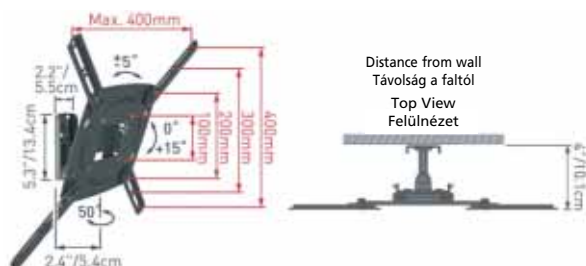
E320 LCD tv tartó 2 funkció LCD tv mount 2 functions
